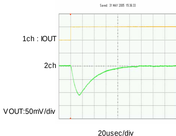
IO UT =1mA → 100mA
