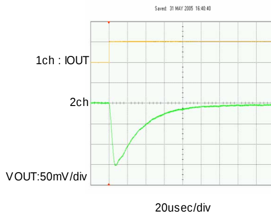
IO UT =1mA → 300mA
