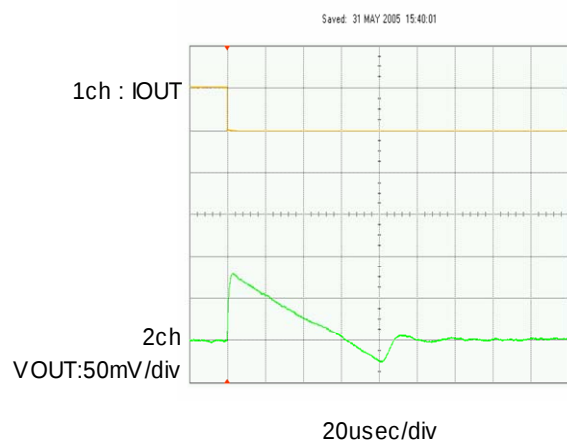
IO UT =100mA → 1mA
