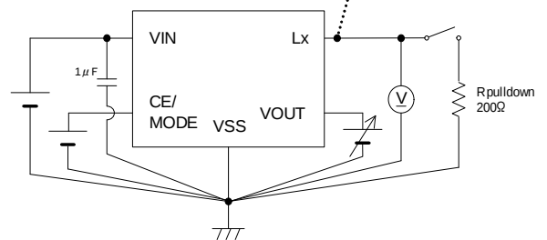
Circuit④
