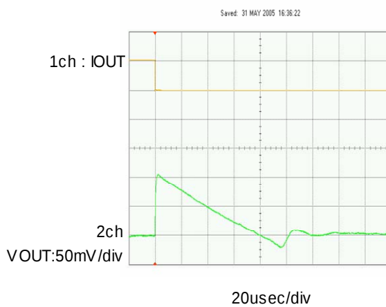
IO UT =300mA → 1mA
