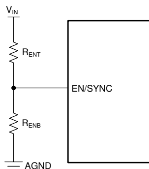
Figure 33. UVLO Using EN
